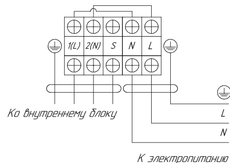
Клеммный терминал наружного блока
