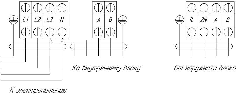
Клеммный терминал наружного блока
