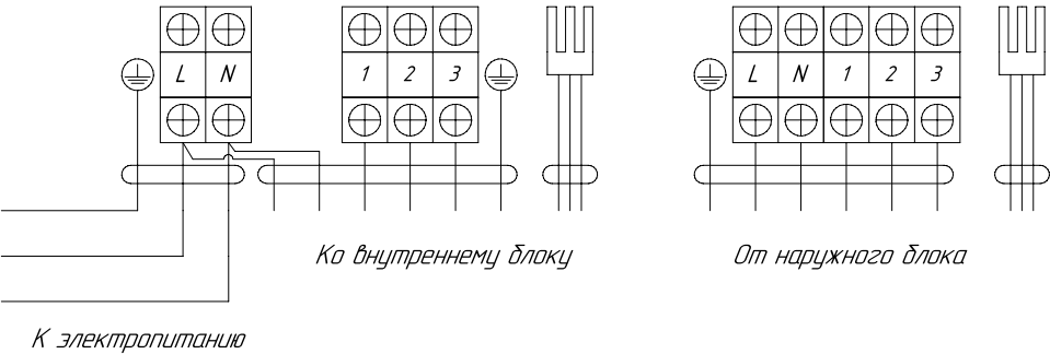
Клеммный терминал наружного блока
